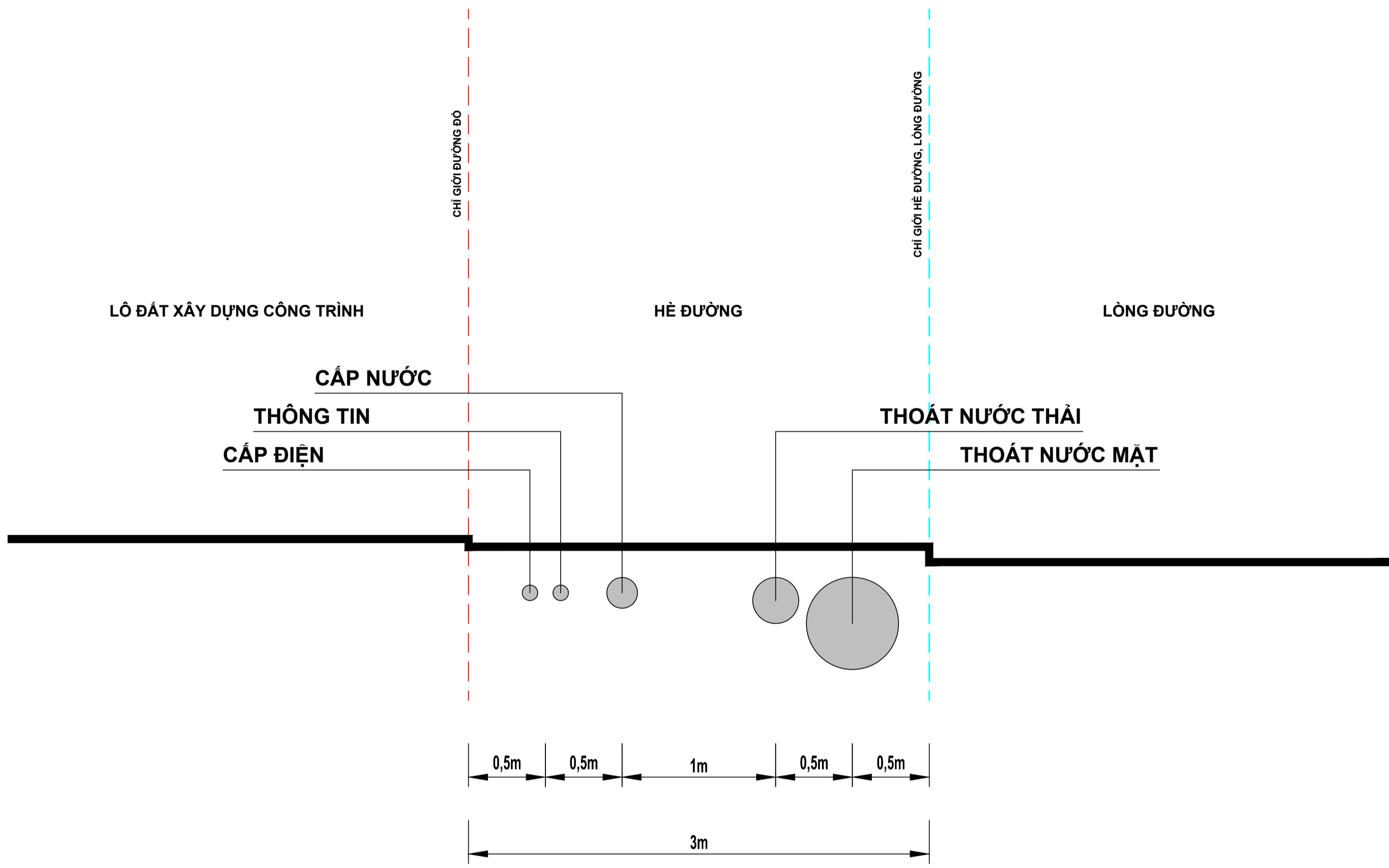
KHOẢNG CÁCH LẮP ĐẶT GIỮA CÁC ĐƯỜNG DÂY, ĐƯỜNG ỐNG ĐI NGẦM
